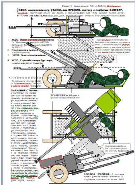
N73/108 Станок для снятия оруж.БМП
