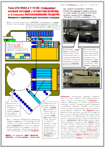
N58/99 Танк Т-72. 2 мех.заряжания
