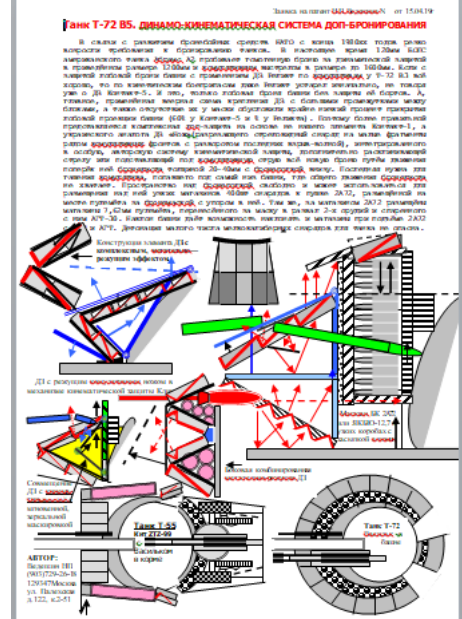
N63/99 ДинамоКинемат.броня Дупль
