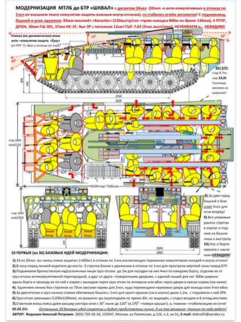
N21/108 МТЛБ. (Проект Ведешина)
