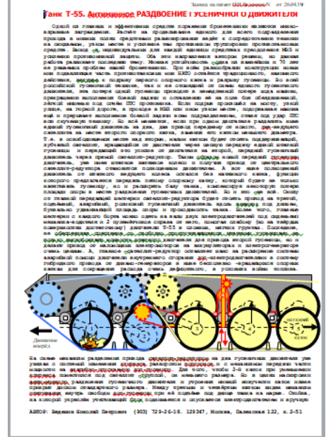
N60/99 Т55/Т-72. Раздвоен.гусениц
